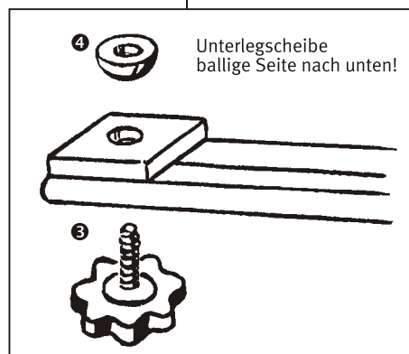
Montage Auszugmechanik
